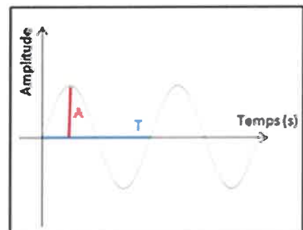
Figure 2. Représentation d'un son simple (son pur)
